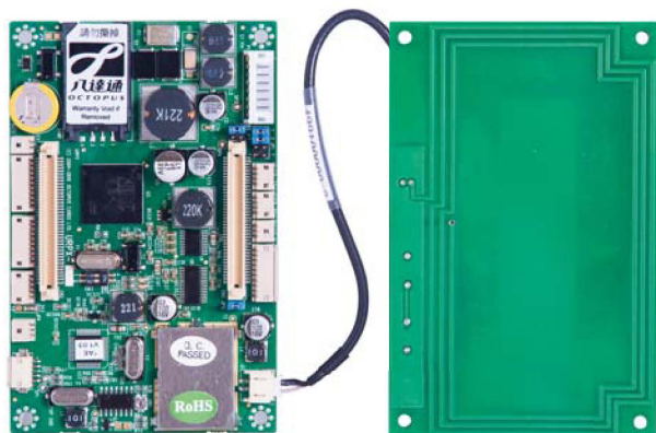
主板及天線
