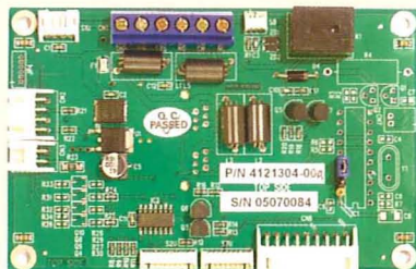
出入保安系統銜接底板
